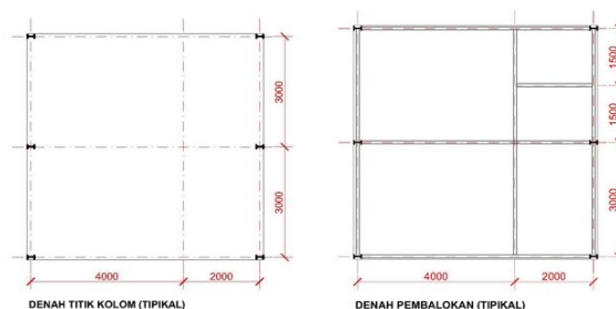
Gambar 12. Semua elemen struktur utama menggunakan baja WF 150 x 75 mm
