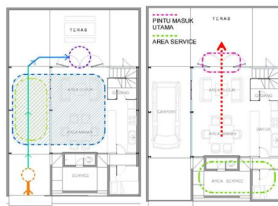
Gambar 6. Pola Sirkulasi dan Orientasi ruang yang tercipta akibat peletakan pintu utama dibelakang
