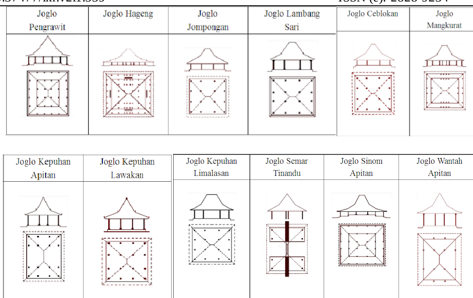
Gambar 1. Jenis Bentuk Atap Joglo (Sumber: Rosiana Andreyani dkk, 2020)
