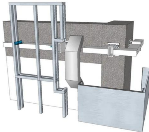
Gambar 4. Detail Rangka ACP (Sumber: analisis pribadi, 2024)
