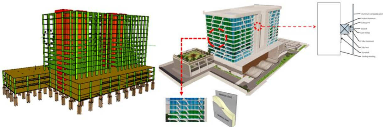
Gambar 5. Penerapan Secondary Skin (Sumber: analisis pribadi, 2023)
