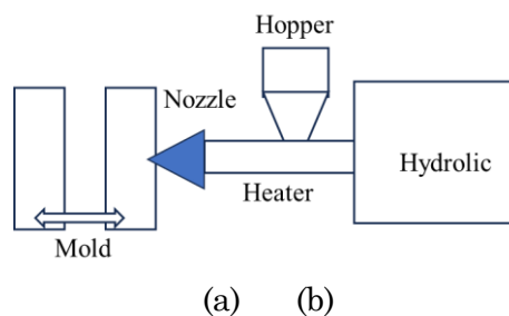
Gambar 2 Mesin Injeksi (a) bagian-bagian utama Mesin Injeksi (b)Tampak atas Mesin rotary 2 injektor
